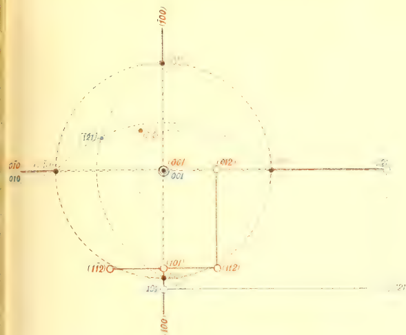
5. Трехосный.
